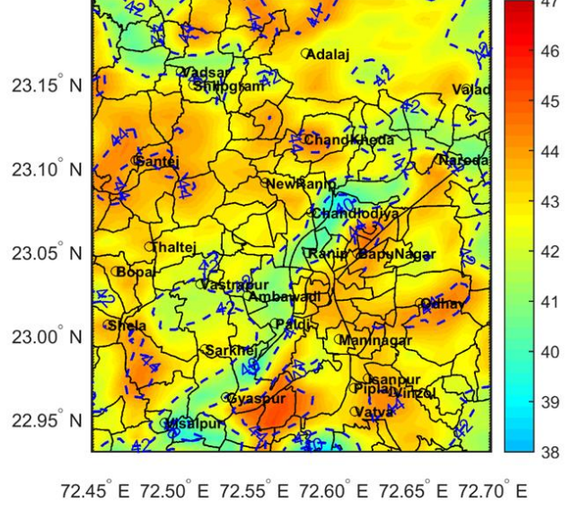
Temperature Forecast for Ahmedabad 17:30 IST 26 May,2023
