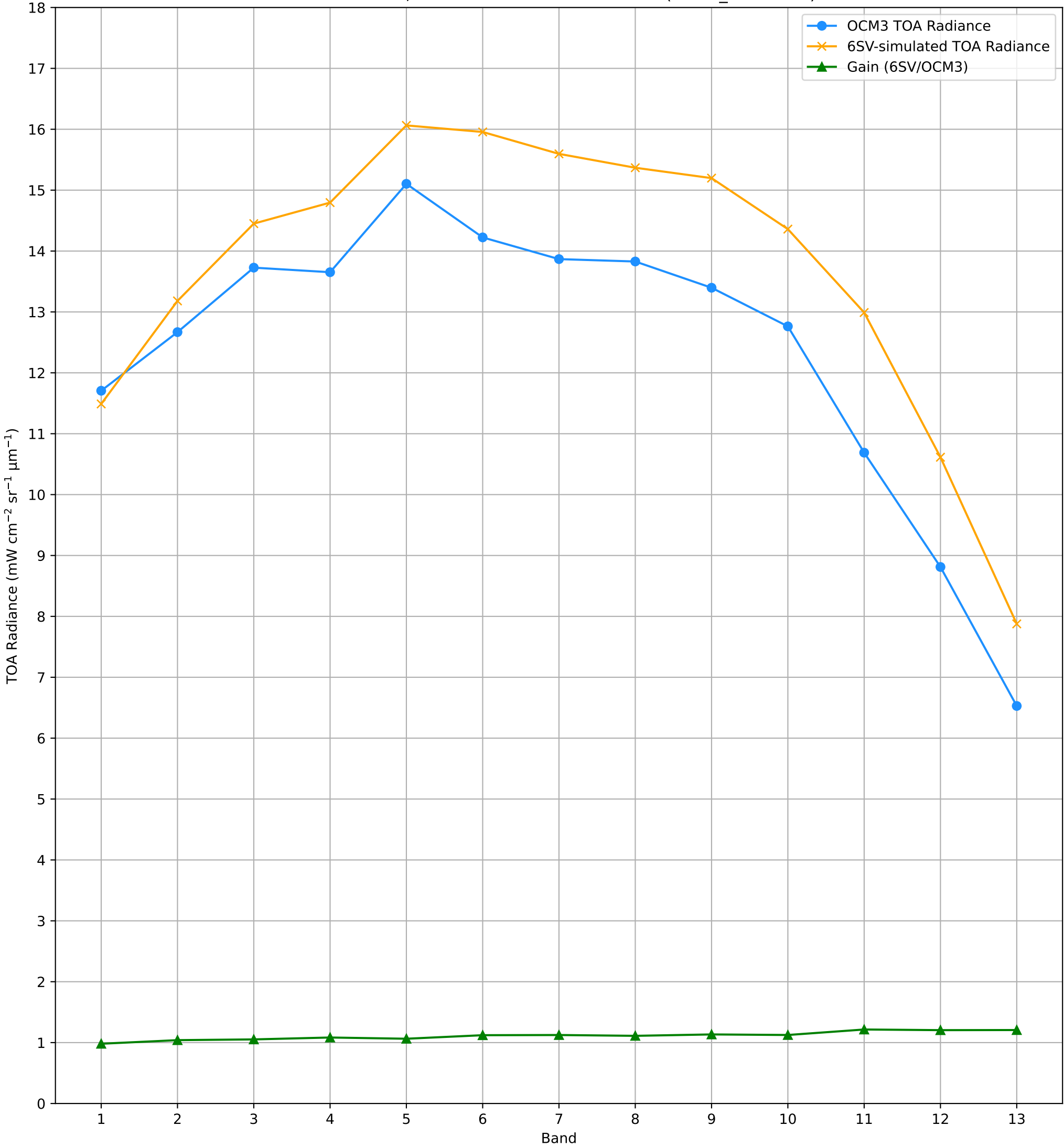
TOA Radiance (OCM3 vs. 6SV) over RVUS RadCalNet Site Lat: 38.497°, Lon: -115.69° - 25-AUG-2026 (STRIP_ID: 19792)
