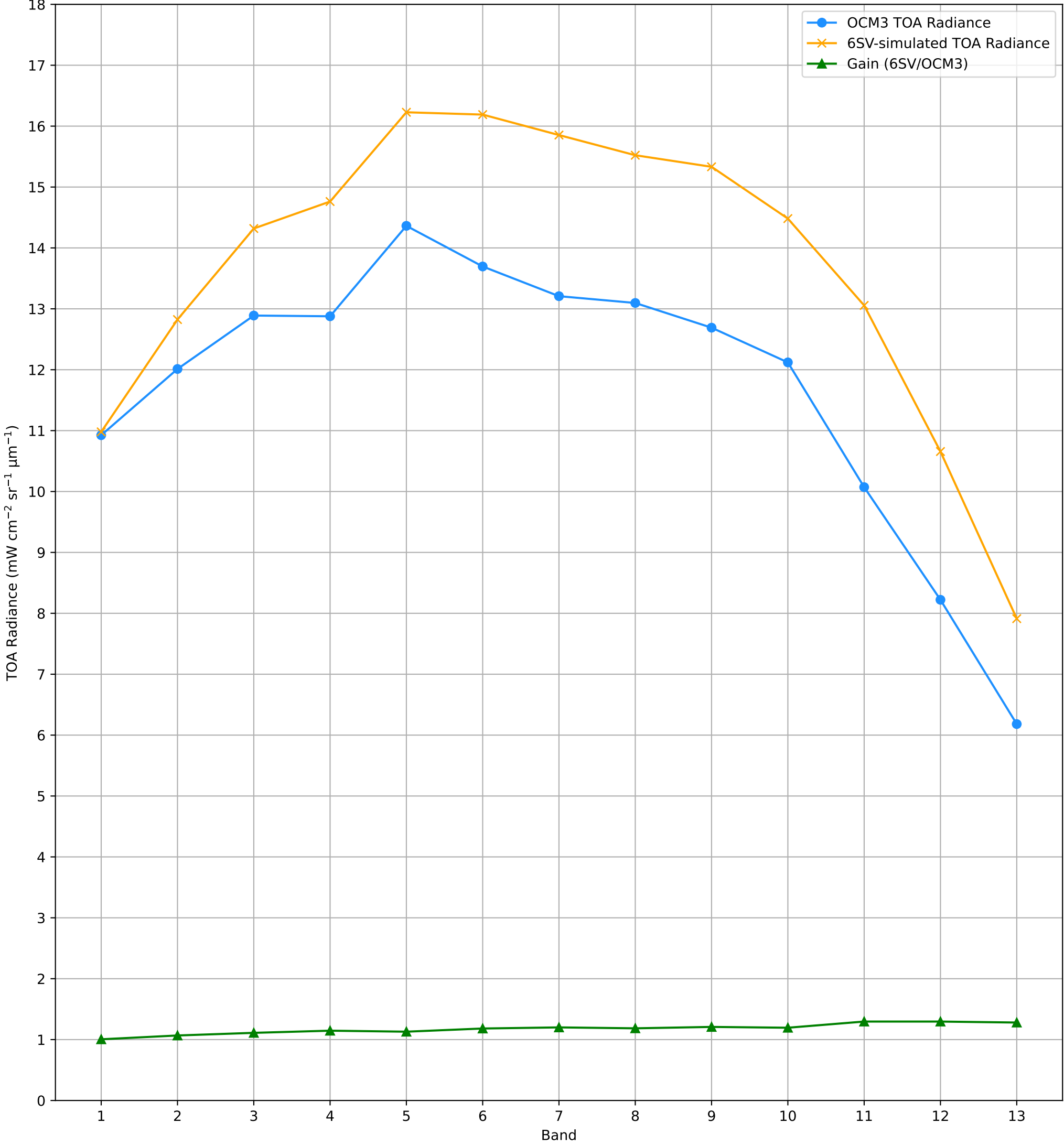
TOA Radiance (OCM3 vs. 6SV) over RVUS RadCalNet Site Lat: 38.497°, Lon: -115.69° - 20-AUG-2026 (STRIP_ID: 19720)
