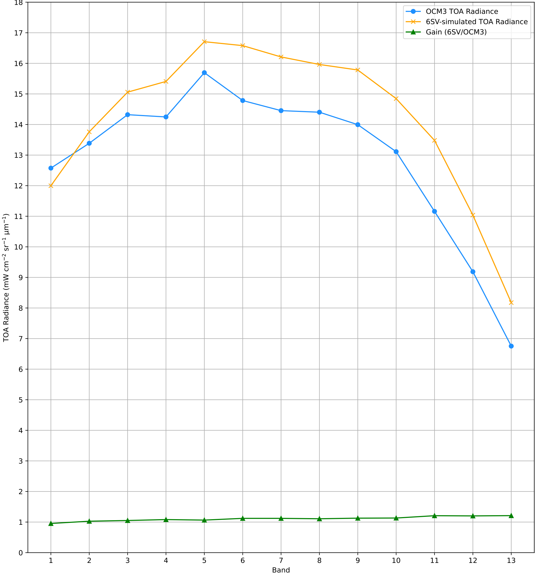
TOA Radiance (OCM3 vs. 6SV) over RVUS RadCalNet Site Lat: 38.497°, Lon: -115.69° - 12-AUG-2026 (STRIP_ID: 19604)
