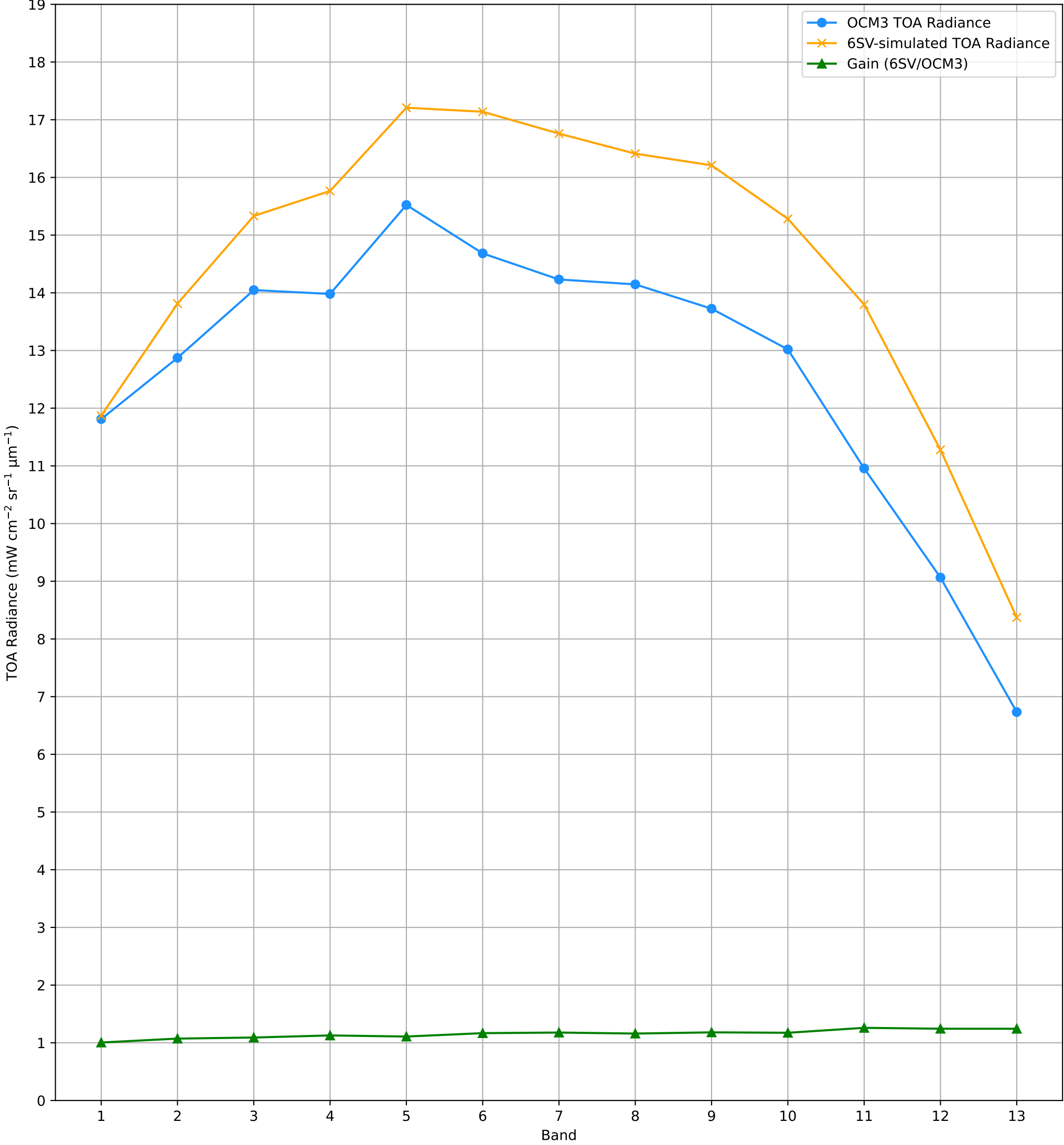
TOA Radiance (OCM3 vs. 6SV) over RVUS RadCalNet Site Lat: 38.497°, Lon: -115.69° - 09-AUG-2026 (STRIP_ID: 19561)
