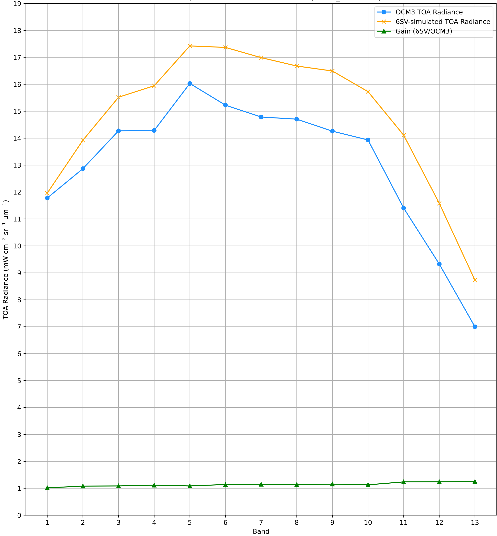
TOA Radiance (OCM3 vs. 6SV) over RVUS RadCalNet Site Lat: 38.497°, Lon: -115.69° - 01-AUG-2026 (STRIP_ID: 19445)
