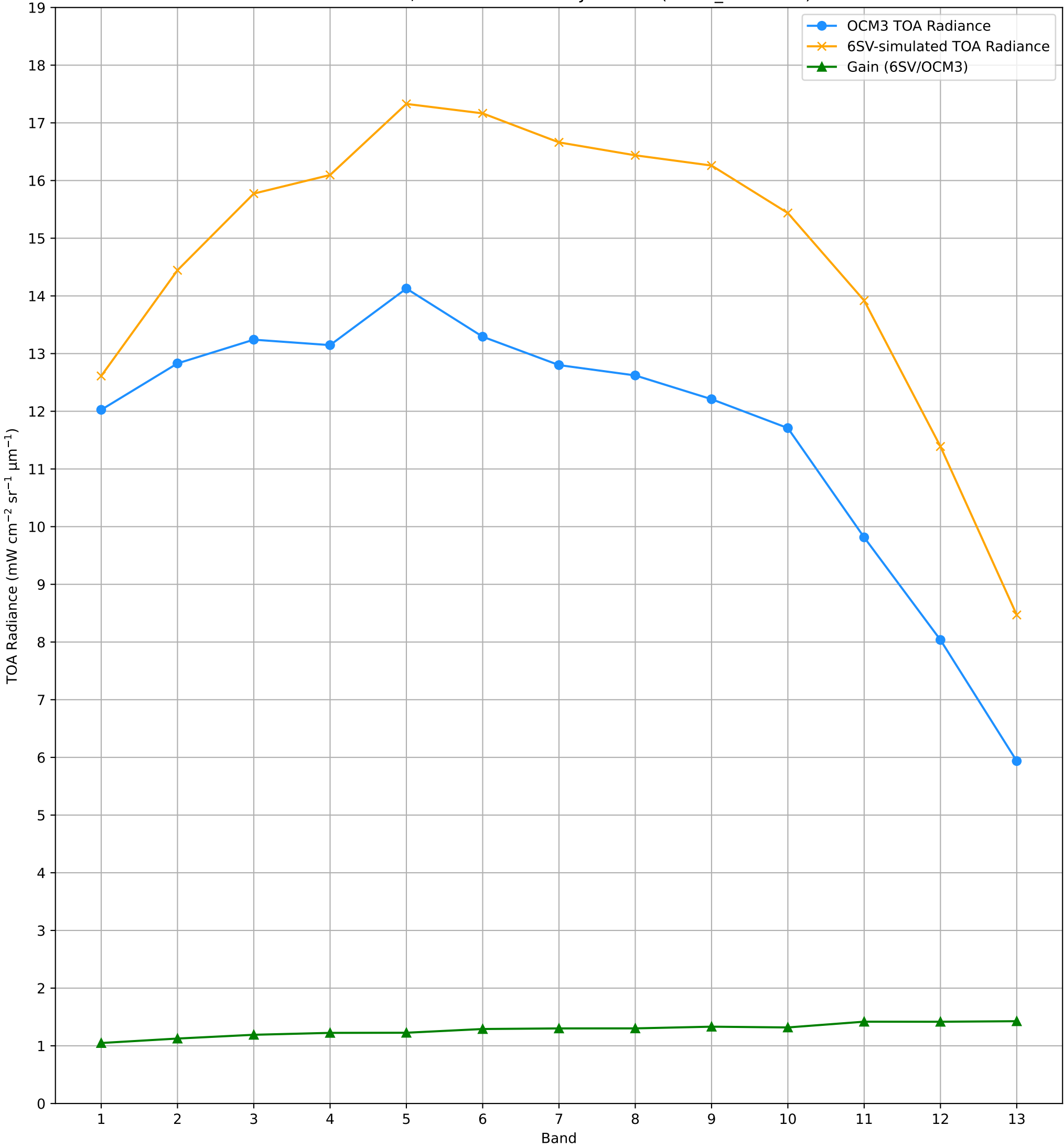
TOA Radiance (OCM3 vs. 6SV) over RVUS RadCalNet Site Lat: 38.497°, Lon: -115.69° - 28-JUL-2026 (STRIP_ID: 19387)
