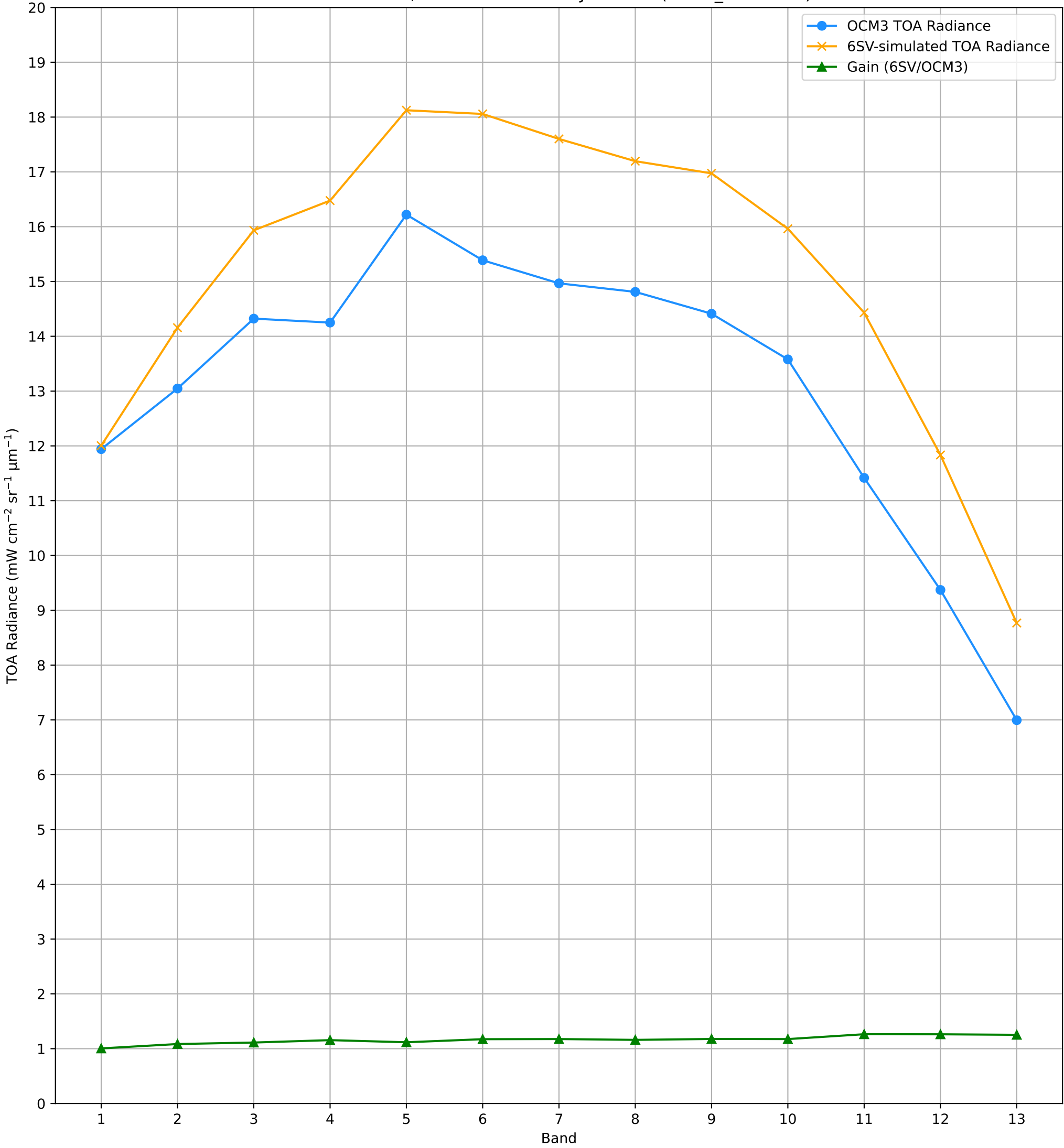
TOA Radiance (OCM3 vs. 6SV) over RVUS RadCalNet Site Lat: 38.497°, Lon: -115.69° - 25-JUL-2026 (STRIP_ID: 19344)
