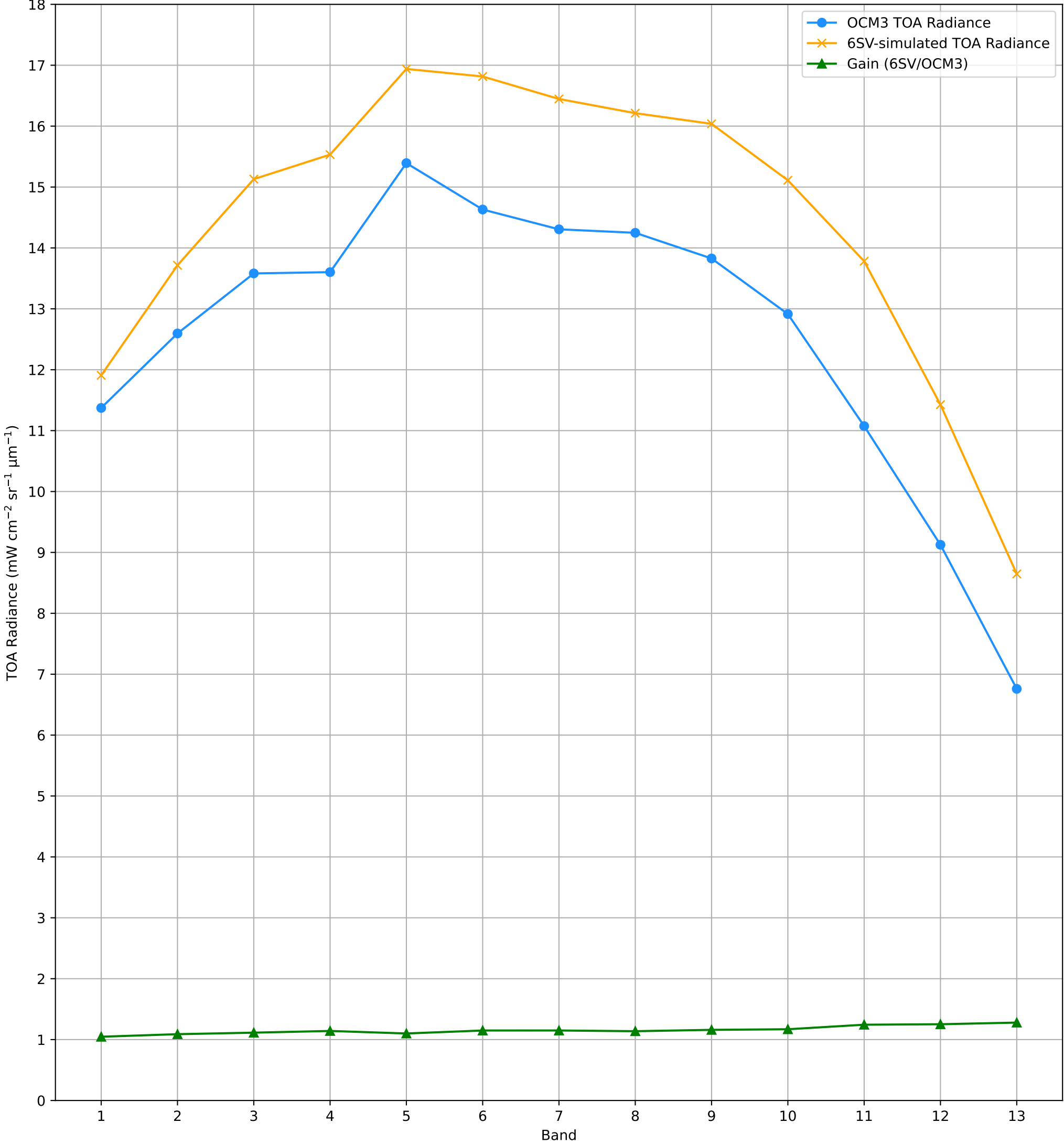
TOA Radiance (OCM3 vs. 6SV) over RVUS RadCalNet Site Lat: 38.497°, Lon: -115.69° - 18-JUL-2026 (STRIP_ID: 19243)
