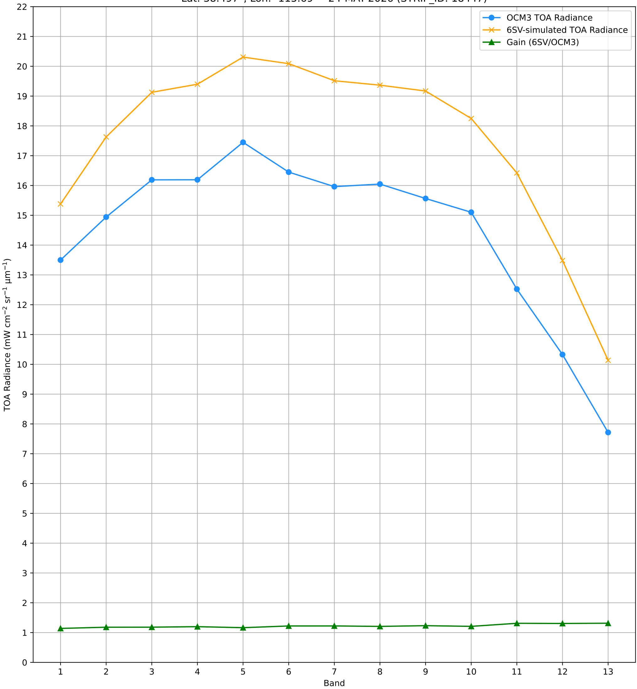
TOA Radiance (OCM3 vs. 6SV) over RVUS RadCalNet Site Lat: 38.497°, Lon: -115.69° - 24-MAY-2026 (STRIP_ID: 18447)
