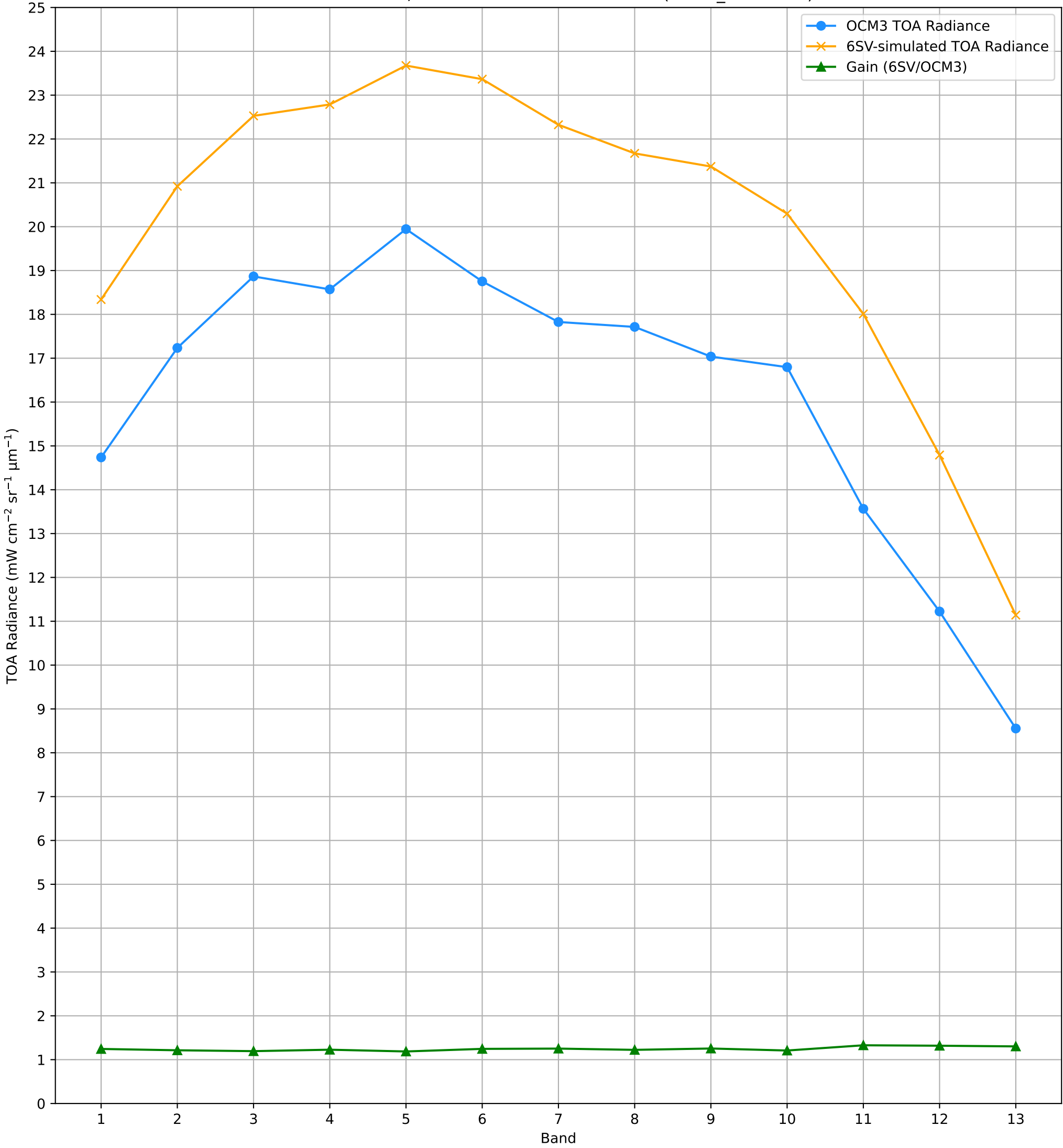
TOA Radiance (OCM3 vs. 6SV) over RVUS RadCalNet Site Lat: 38.497°, Lon: -115.69° - 10-MAY-2026 (STRIP_ID: 18245)
